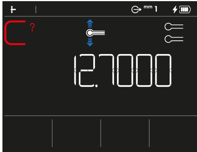
Startbildschirm des Vorgangs zur Taster-Kalibrierung
