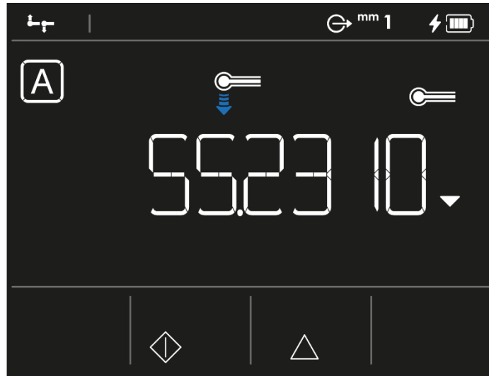
Messergebnis aus einem Antastvorgang nach unten im ST1-Modus.
