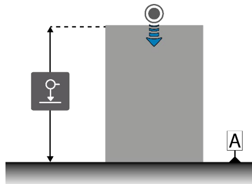
Die indirekte Referenz befindet sich auf Höhe der Hartgesteinsplatte
