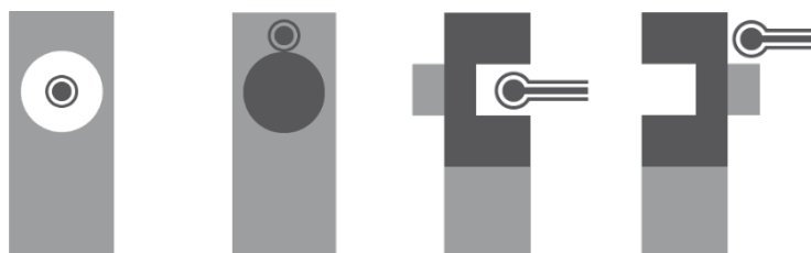
Elemente, bei denen doppeltes Antasten und Messen in zwei Richtungen erforderlich ist: Bohrung, Achse, Nut, Steg
